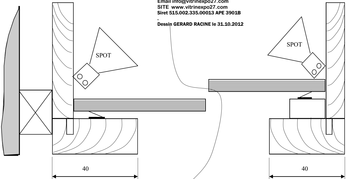
DETAIL EN PLAN position des spots et joints
